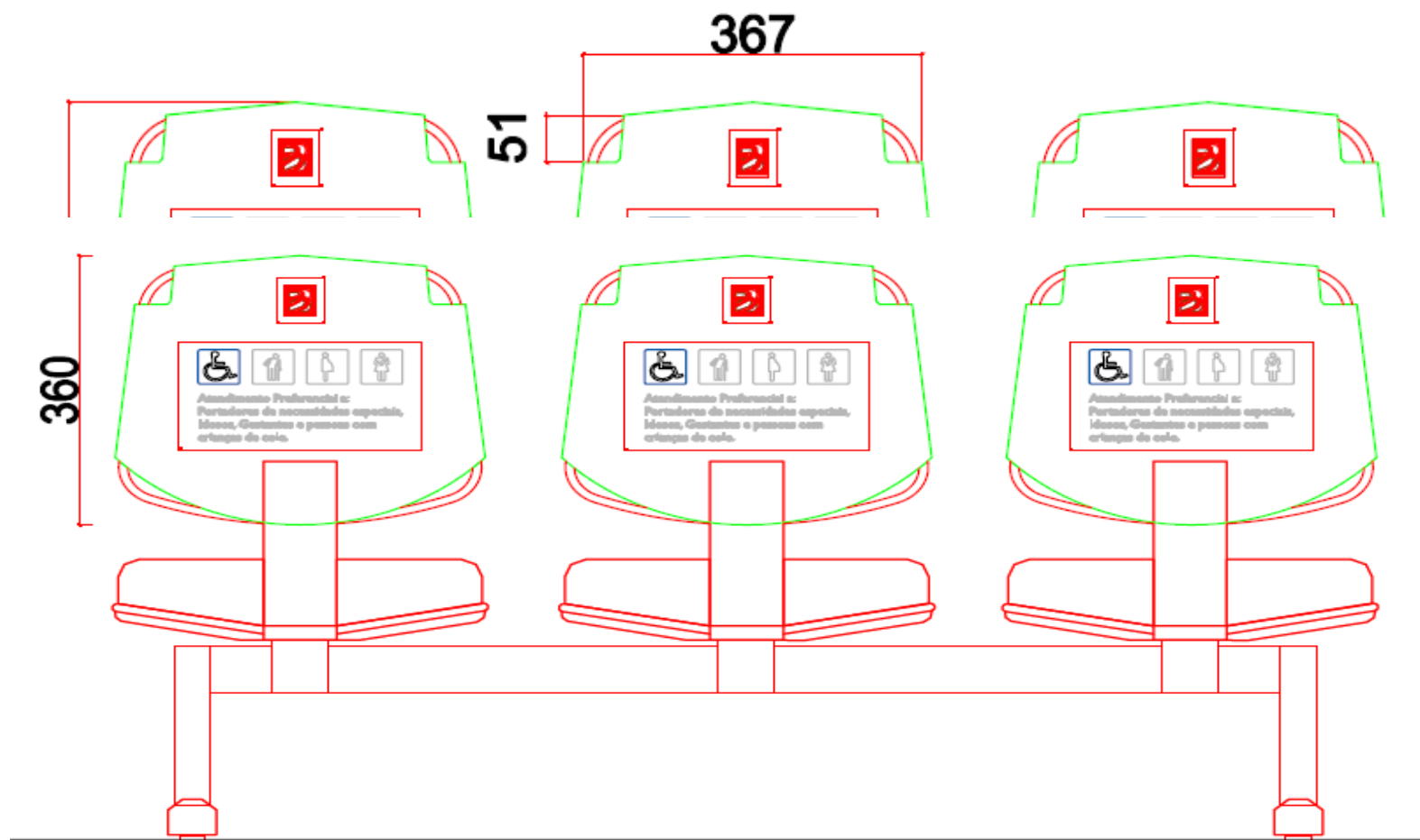
Vista Posterior da Longarina com CLAP
