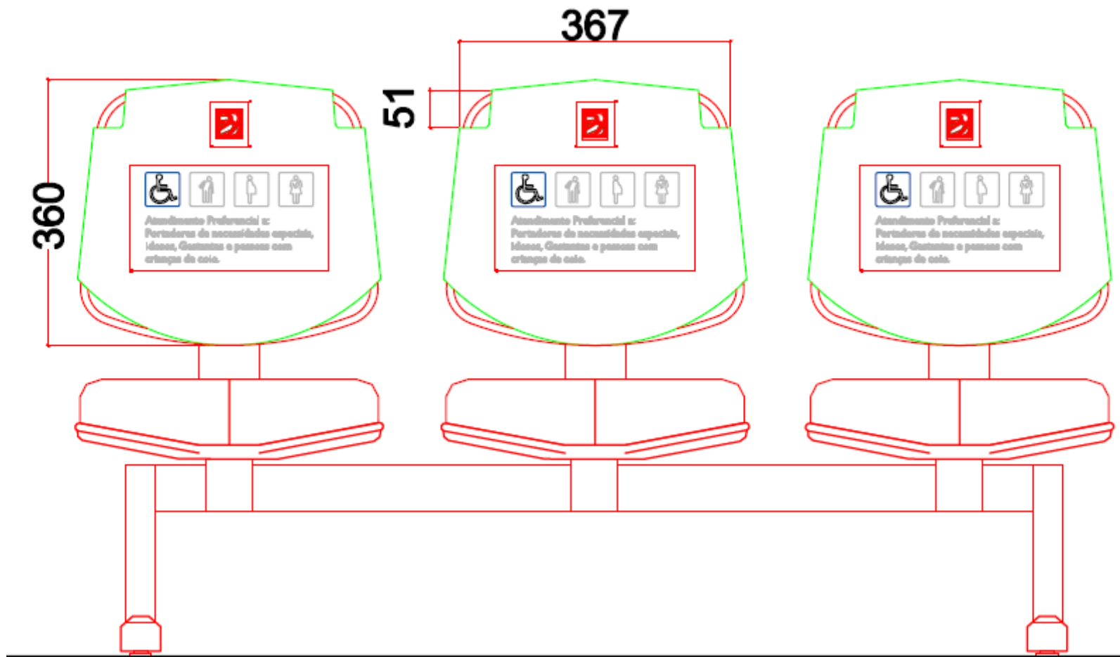
Vista Frontal da Longarina com CLAP
